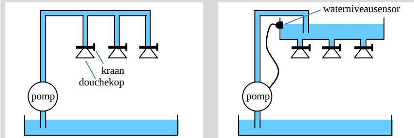
Figuur 13 – Een kampdouches in twee varianten: zonder (links) en met (rechts) voorraadvat.
