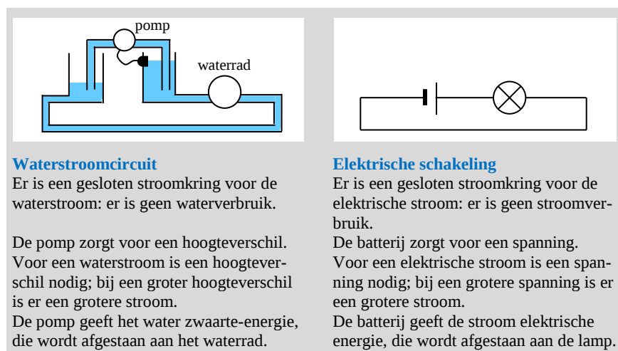
Figuur 19 – In de waterstroomanalogie zijn beide manieren waarop je naar spanning kunt kijken zichtbaar.
